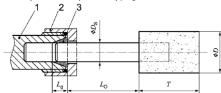
Rys. 1: Długość mocowania uchwyty zaciskowego i zacisku
