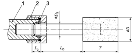
Resim 1: Germe aynası ile germe pensi arasındaki gerdirme uzunluğu
