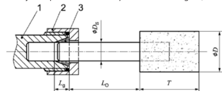
Figura 1: lungimea de încăstrare a mandrinei și clemei de strângere
