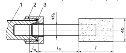
Fig. 1: Inspänningslängd från spännchuck och spännhylsa Förklaring
