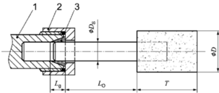
Bild 1: Einspannlänge von Spannutter und Spannange Legende
