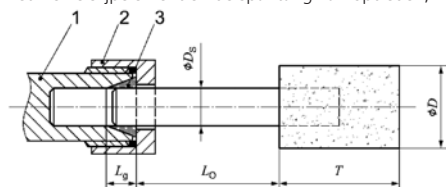
Afbeelding 1: Spanlengte van de spankop en spantang Legenda
