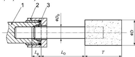
Slika 1: Vpenjalna dolžina vpenjala in vpenjalnih čeljusti Legenda
