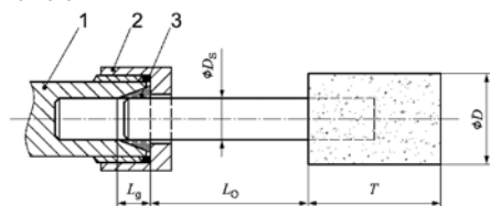
Εικόνα 1: Μήκος τοποθέτησης εργαλειοδέτη και κόλعت Υπόμνημα
