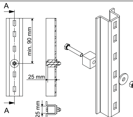
Abb. 12 Feste Endsicherung Steigschutzschiene
